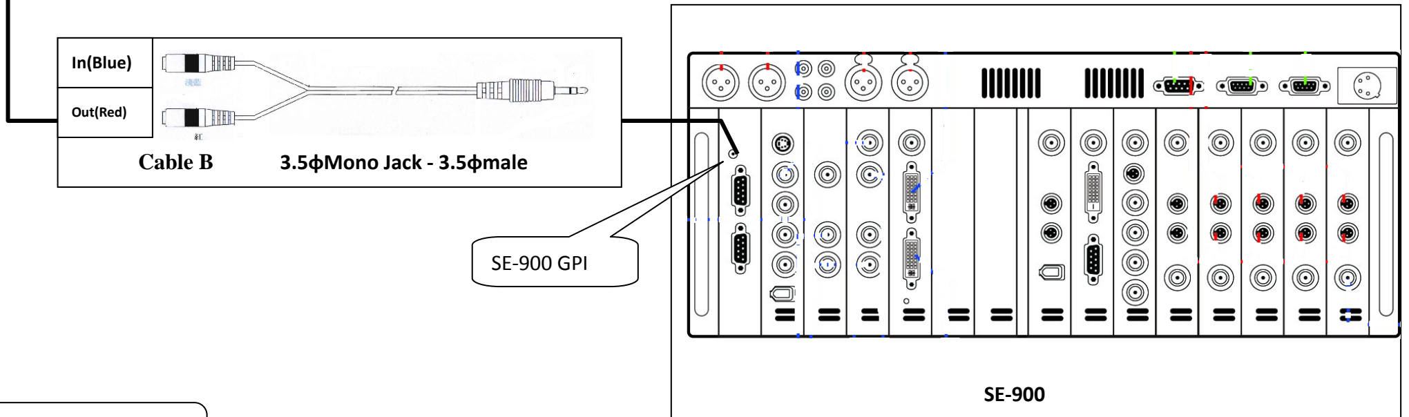
SE-900 / DN-200 GPI Link Map
